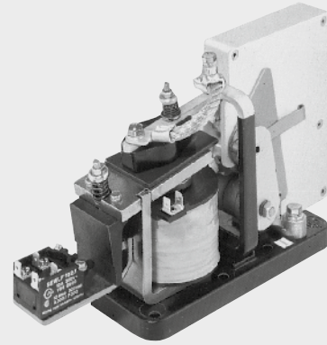
GLA 121 mit Hilfskontakten 1 S/1 Ö GLA 121 with Aux. Contacts 1 NO/1 NC
