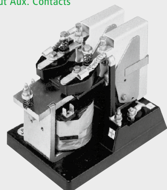
GLA 106 ohne Hilfskontakte GLA 106 without Aux. Contacts
