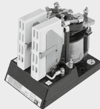
GLA 106 ohne Hilfskontakte GLA 106 without Aux. Contacts
